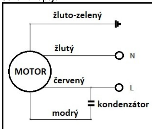
Schéma zapojení
