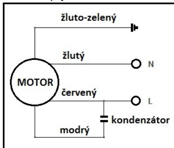
Schéma zapojení
