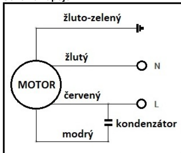
Schéma zapojení
