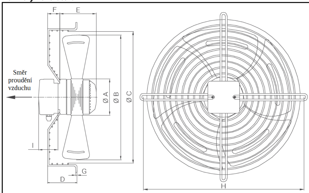
Rozměry ventilátoru
