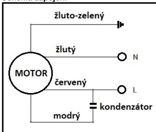
Schéma zapojení
