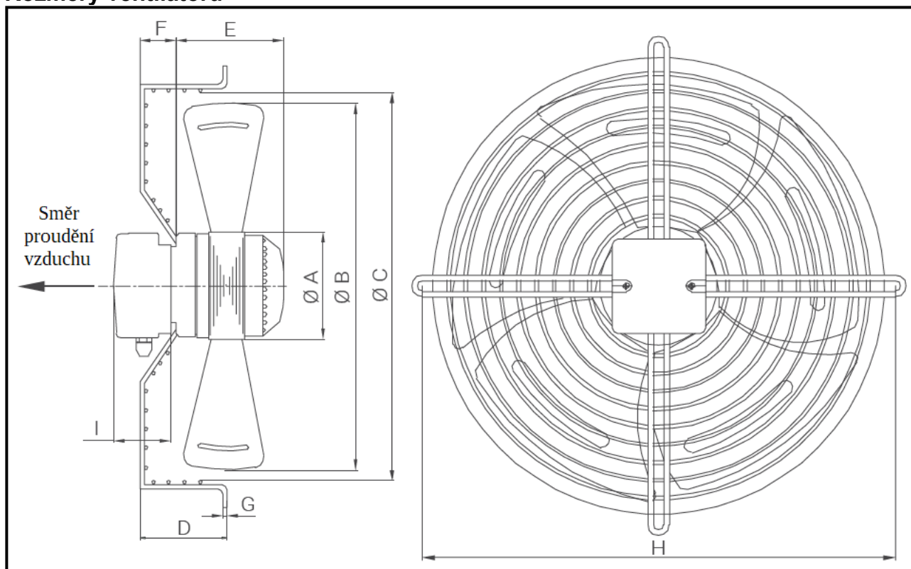
Rozměry ventilátoru
