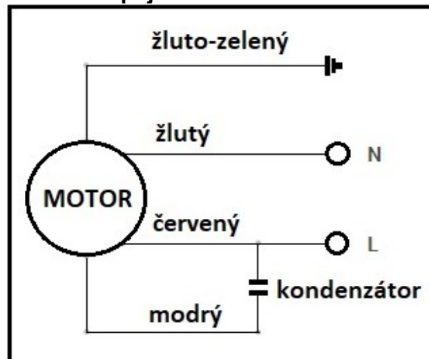
Schéma zapojení
