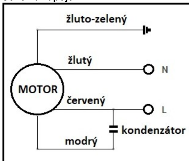
Schéma zapojení
