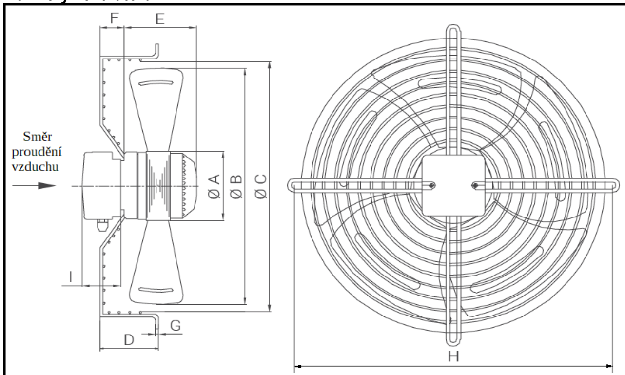
Rozměry ventilátoru
