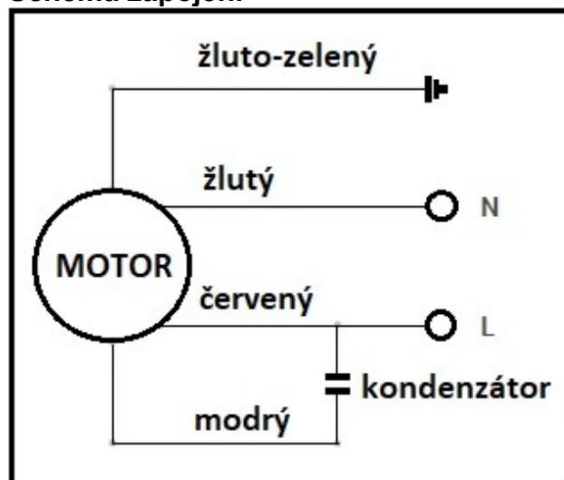
Schéma zapojení
