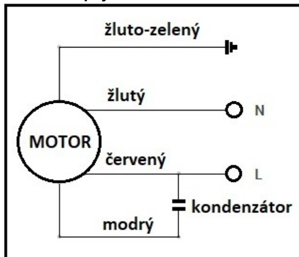
Schéma zapojení
