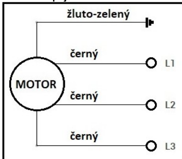
Schéma zapojení
