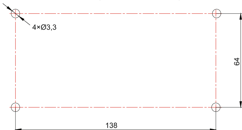
Obr. 3-11: Otvory pro montáž instalační krabice
